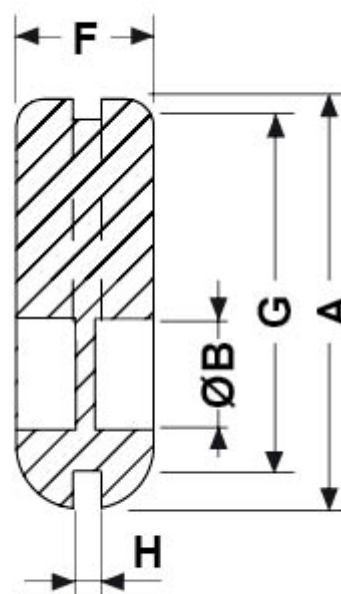
Sez. A-A
